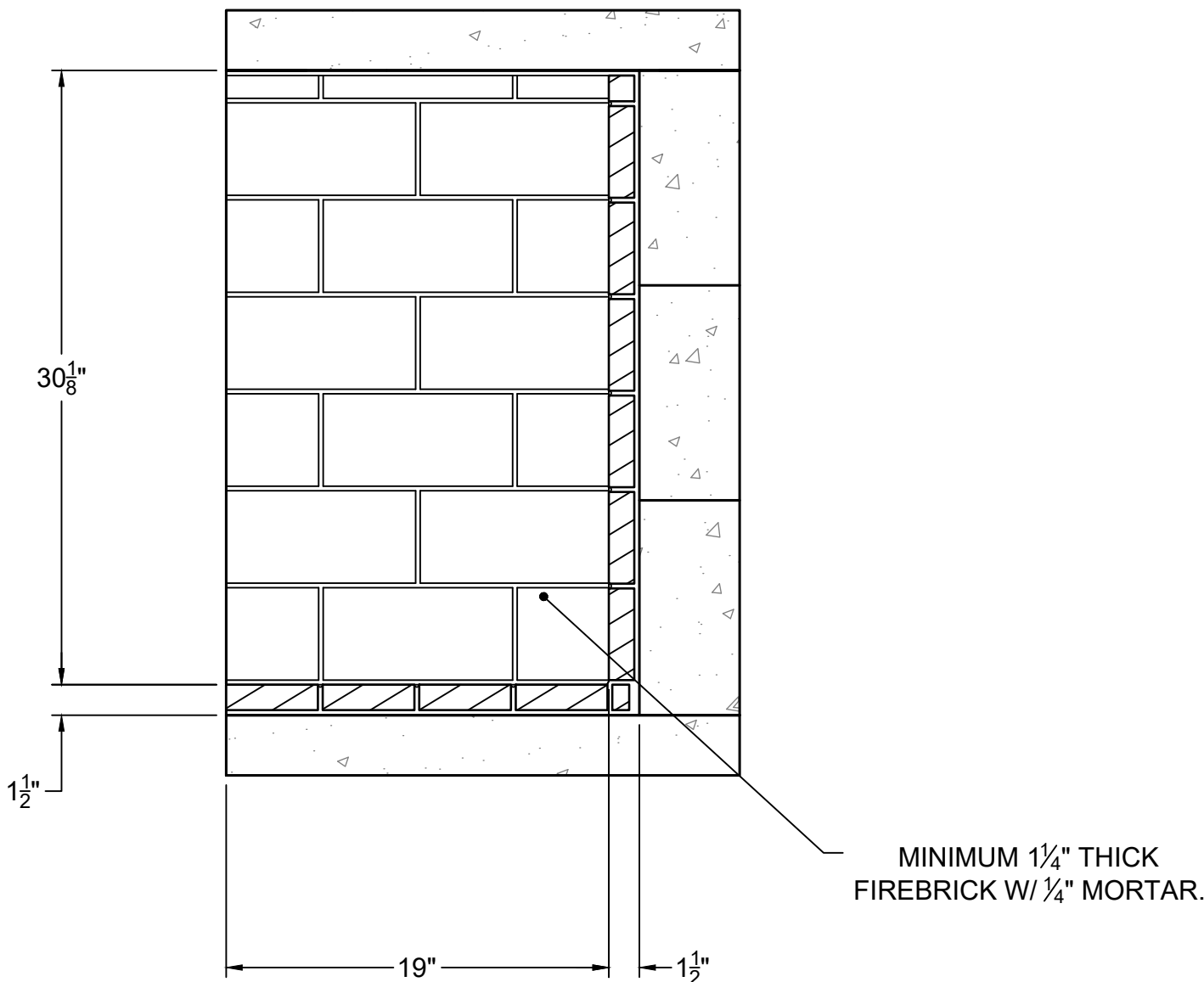
SECTION A-A
