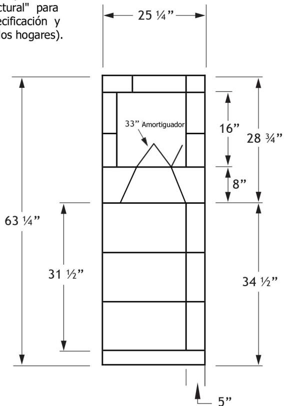
Vista lateral
