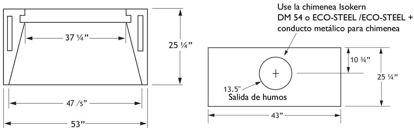
Vista plano
