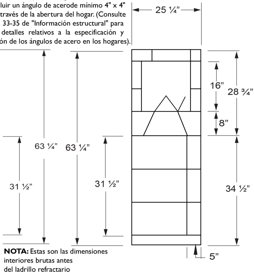
Vista lateral
