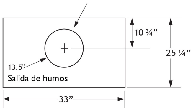
Vista superior
