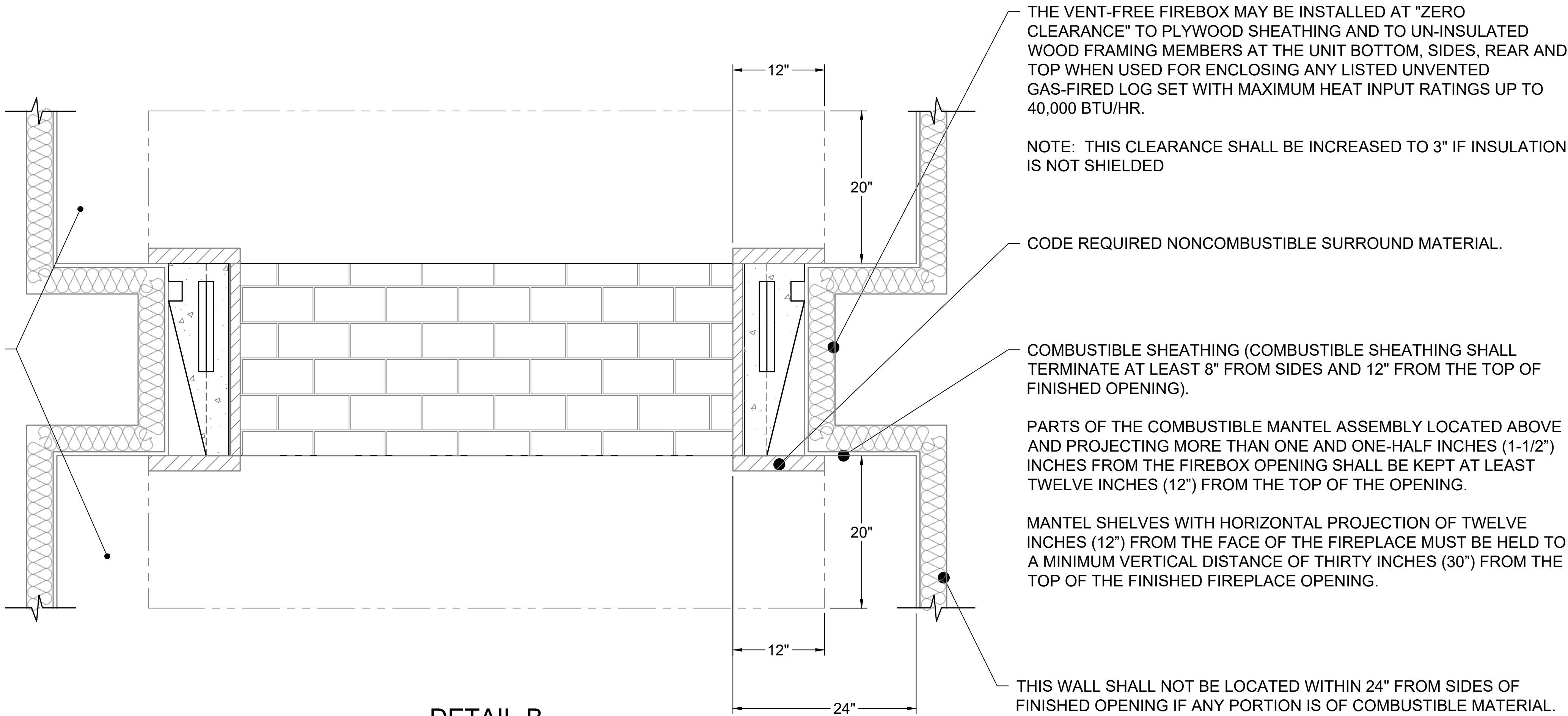
DETAIL-B
