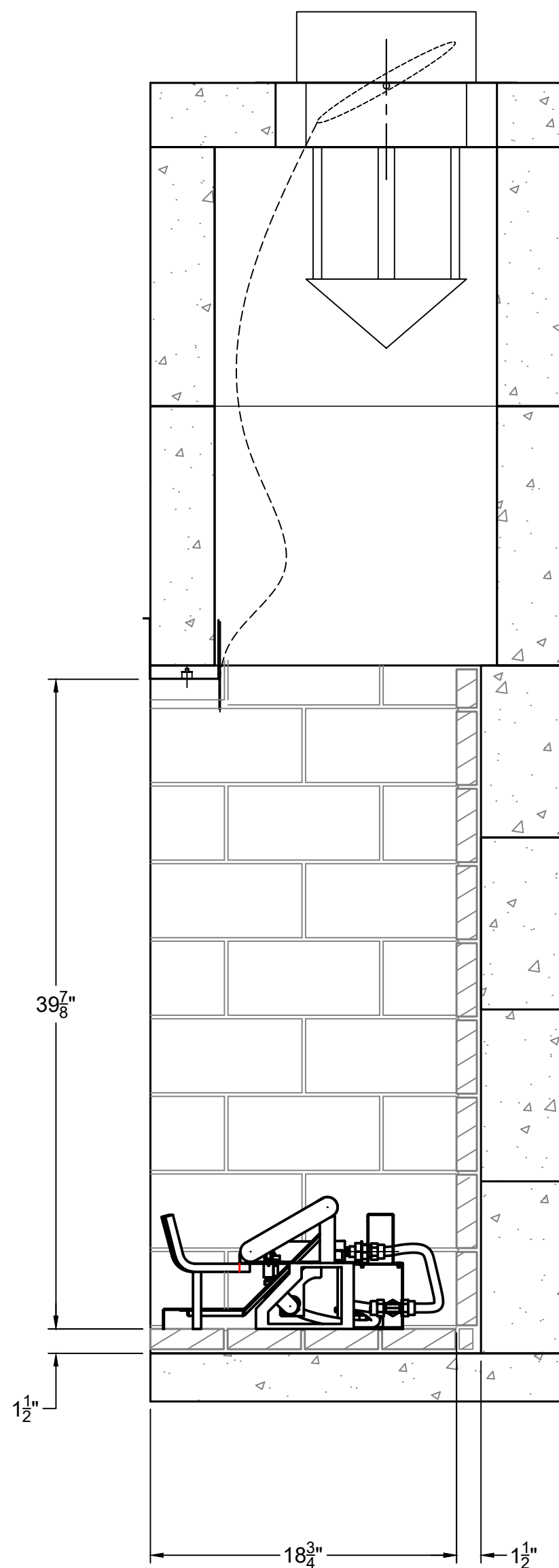
SECTION A-A
