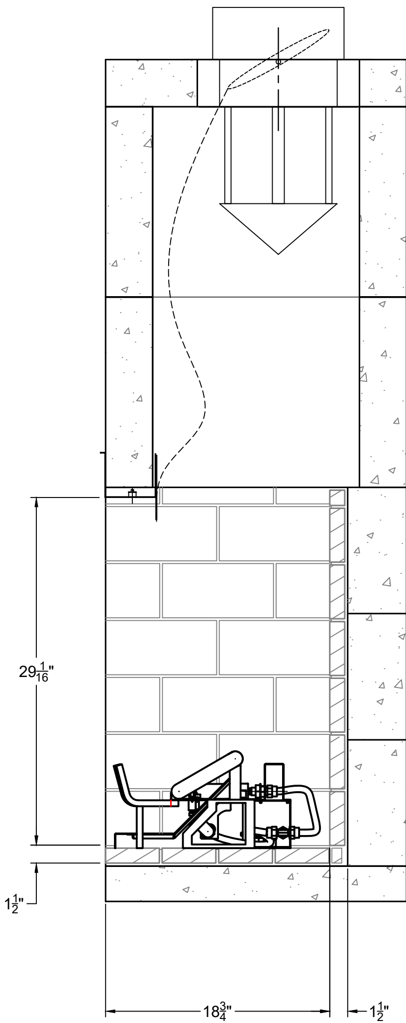
SECTION A-A
