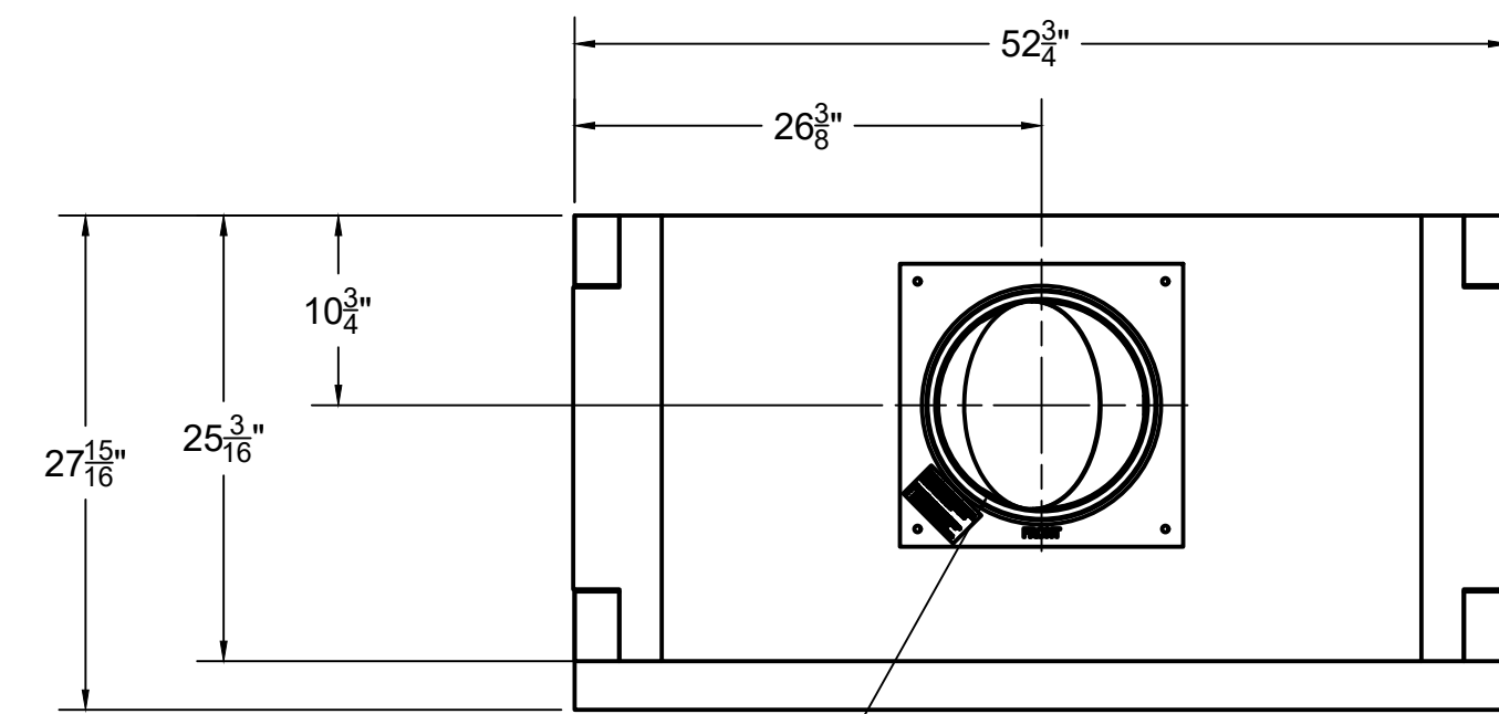
TOP
