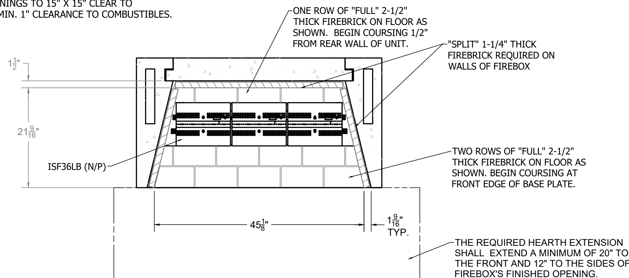
SECTION A-A
