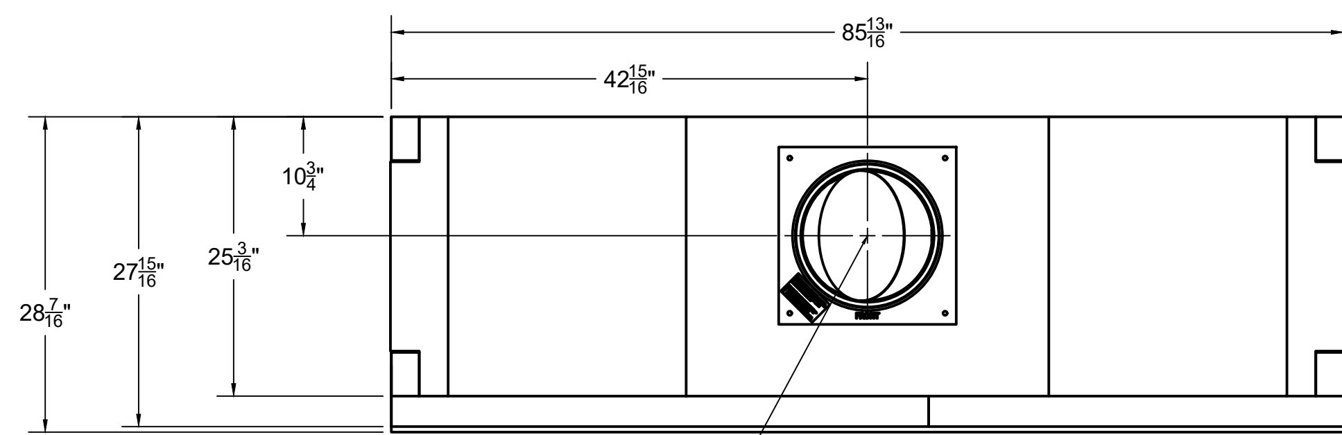
TOP
