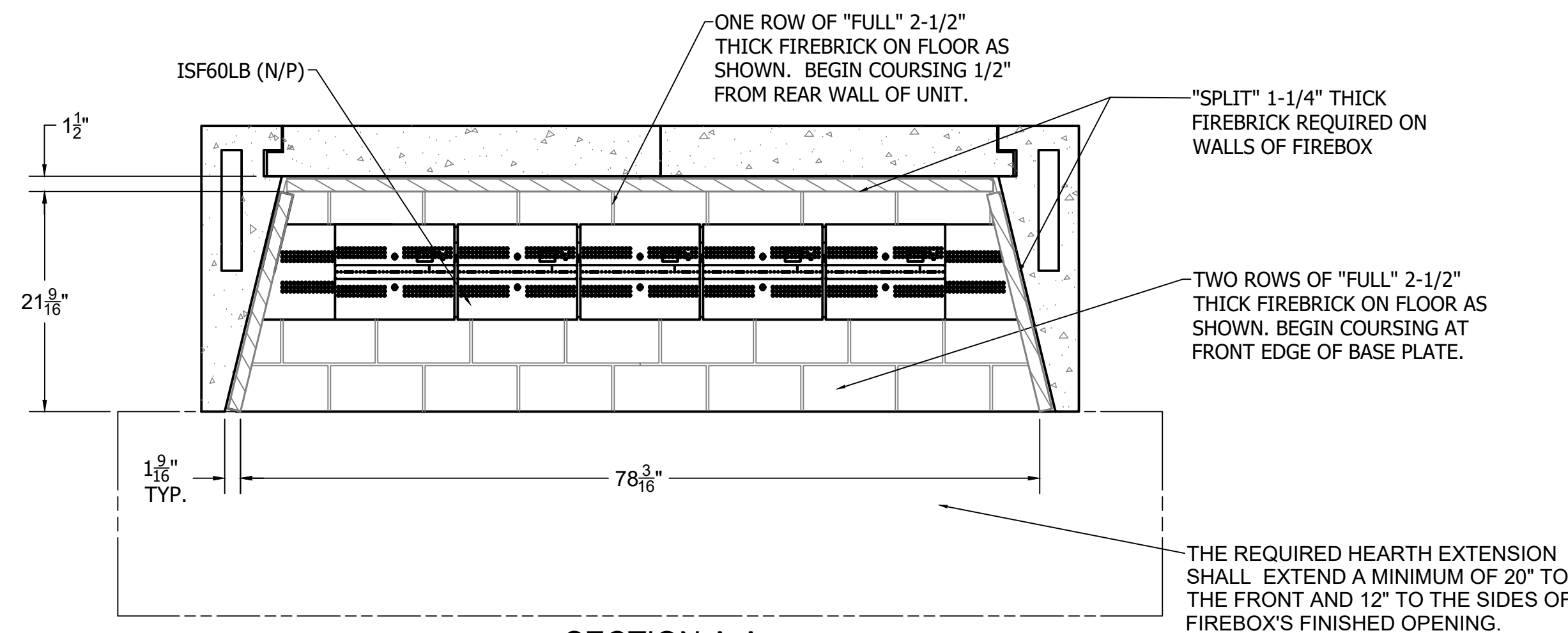
SECTION A-A
