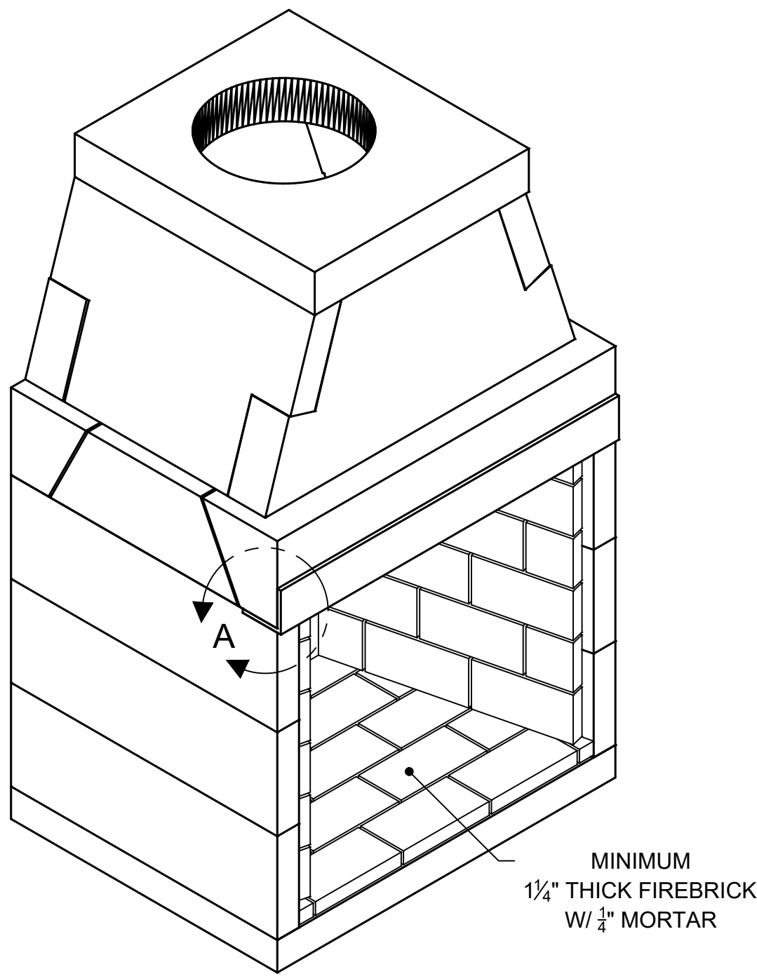
ISOMETRIC VIEW (N.T.S)
