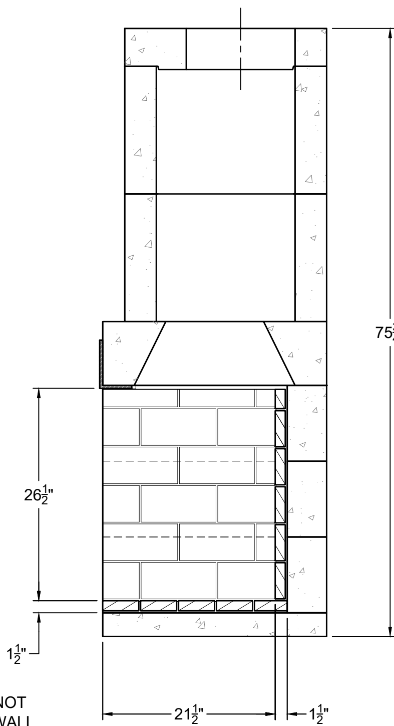
SECTION A-A
