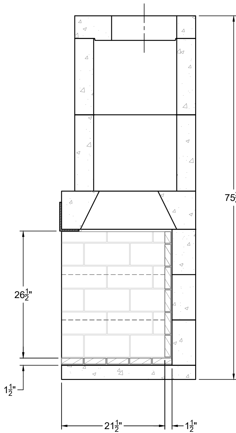
SECTION A-A
